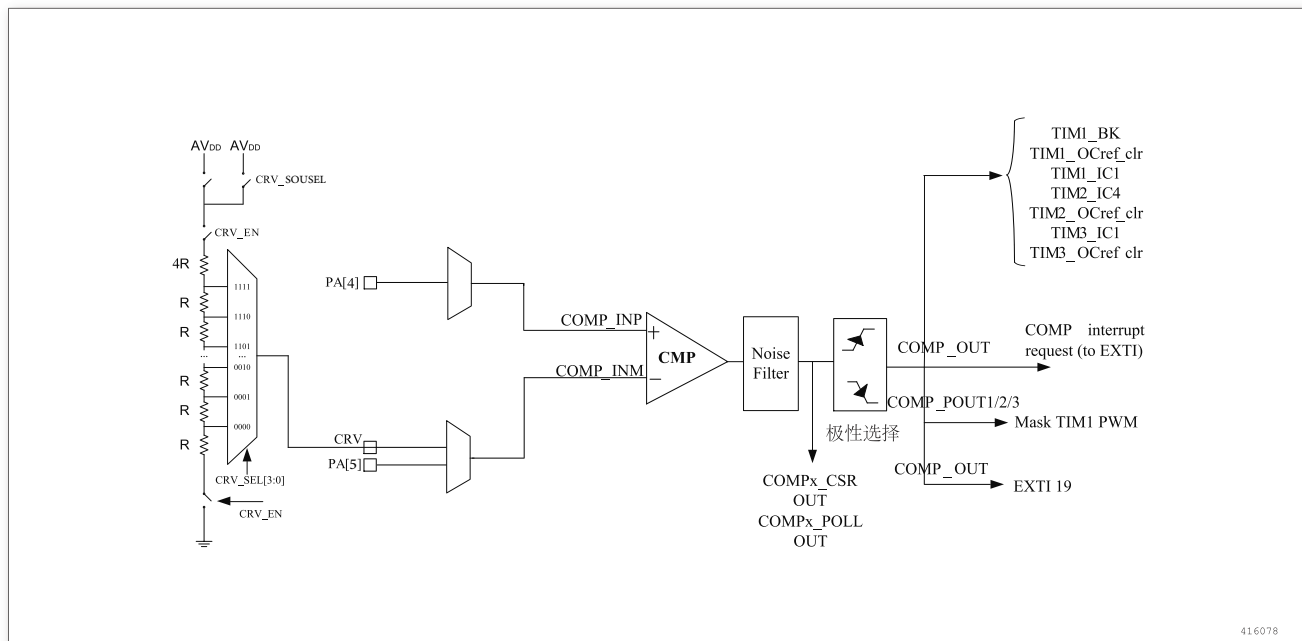
图 29. 比较器框图
