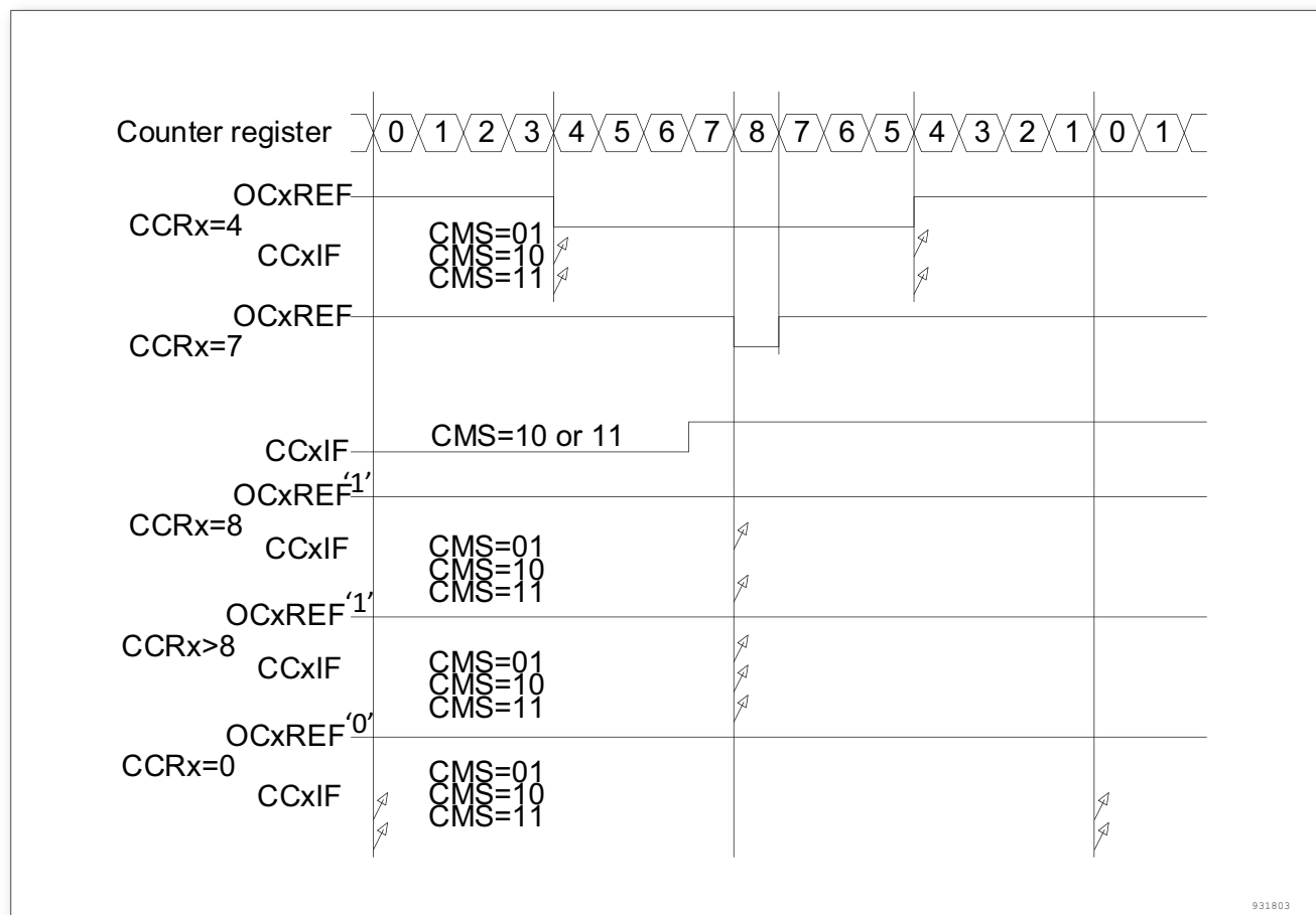
图 64. 中央对齐的 PWM 波形 (ARR = 8)
