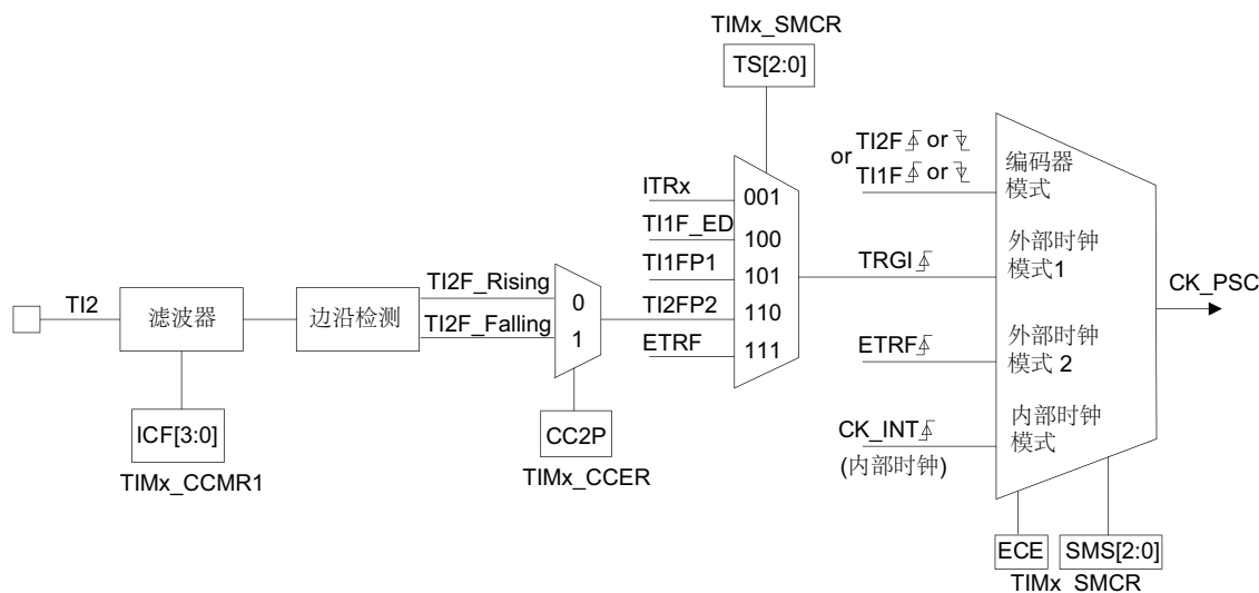
图 53. TI2 外部时钟连接例子
