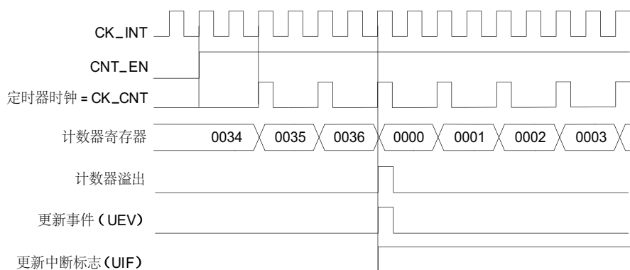
图 175. 计数器时序图, 内部时钟分频因子为 2
