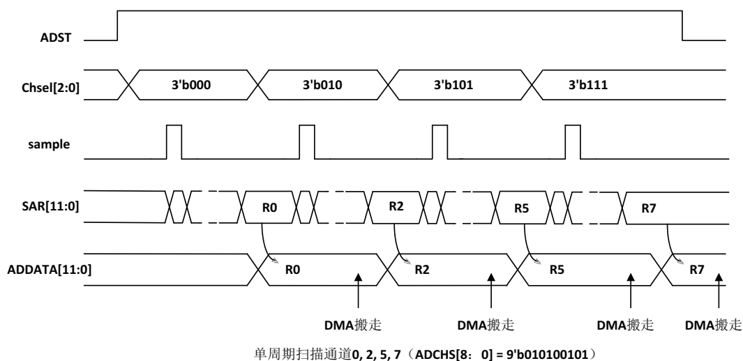
图 26. 单周期扫描下使能通道转换时序图
