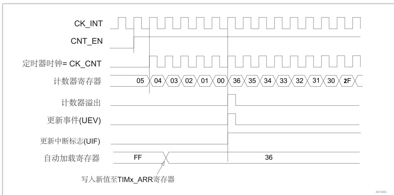
图 92. 计数器时序图，当没有使用重复计数器时的更新事件
