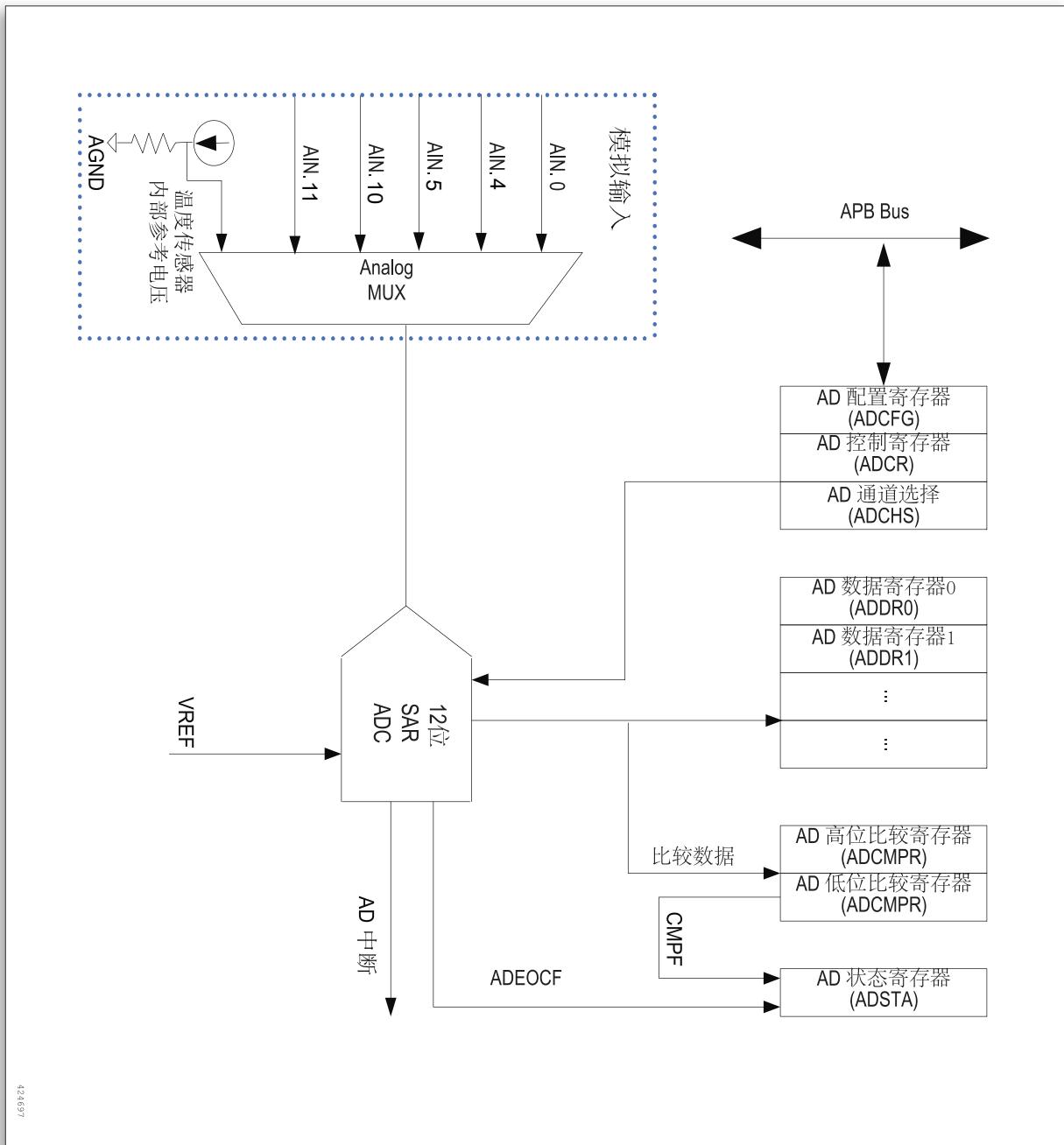
图 24. ADC 框图
