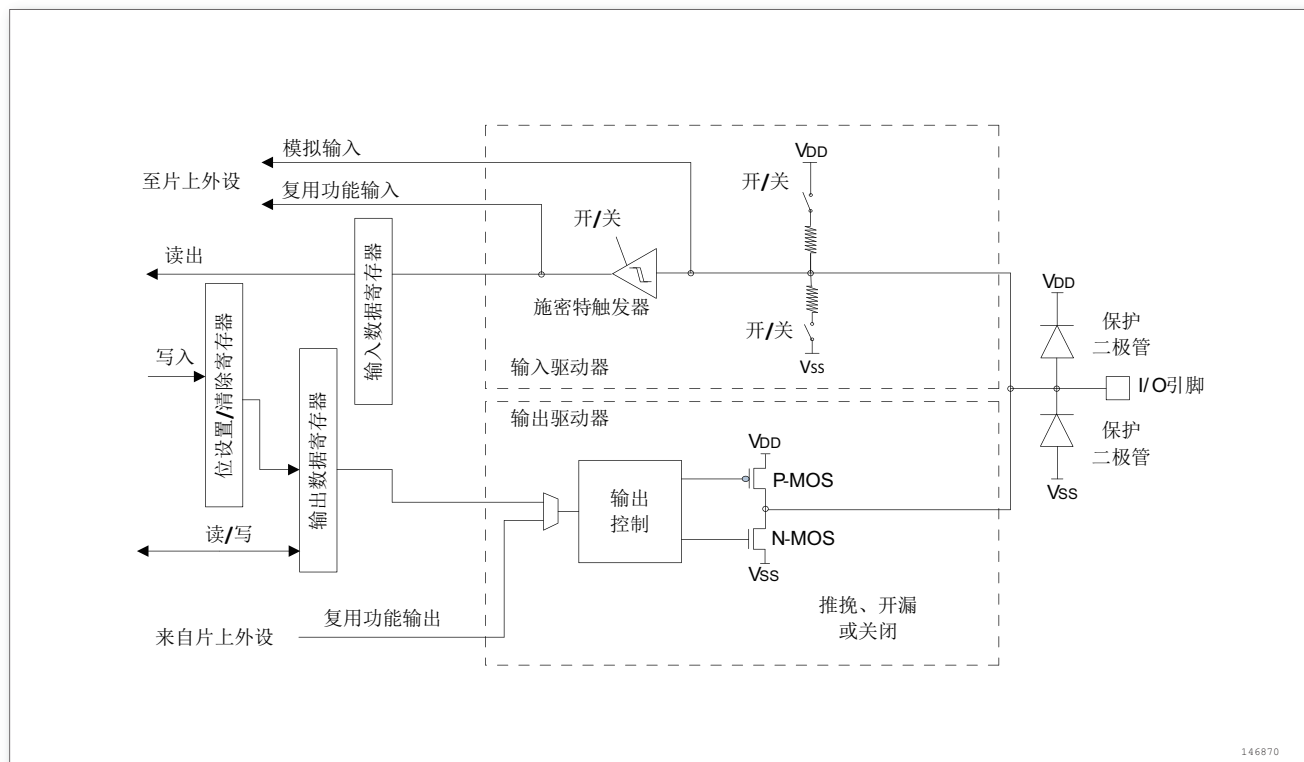
图 15. I/O 端口位的基本结构
