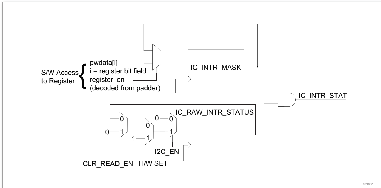
图 226. 中断机制
