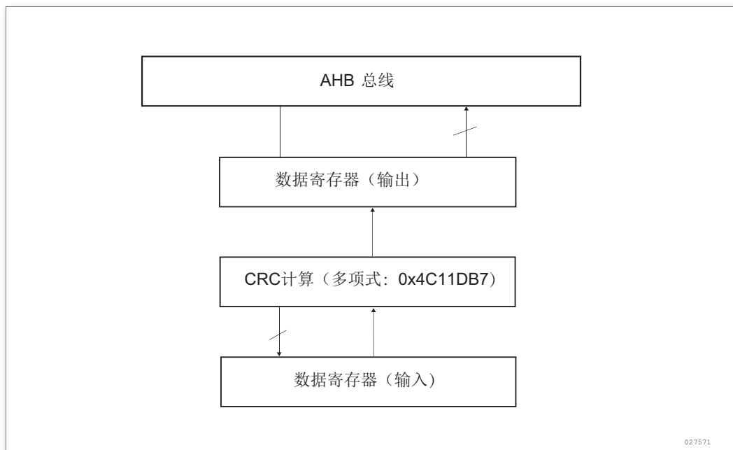
图 10. CRC 计算单元框图
