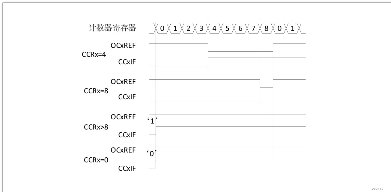
图 201. 边沿对齐的 PWM 波形 (ARR = 8)
