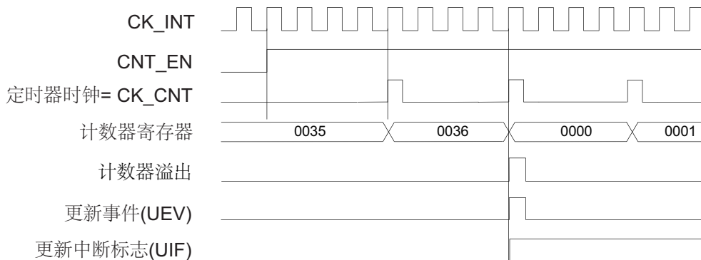
图 176. 计数器时序图, 内部时钟分频因子为 4
