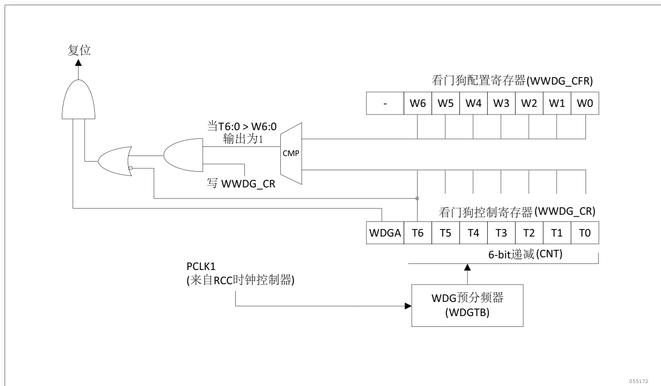
图 208. 看门狗框图
