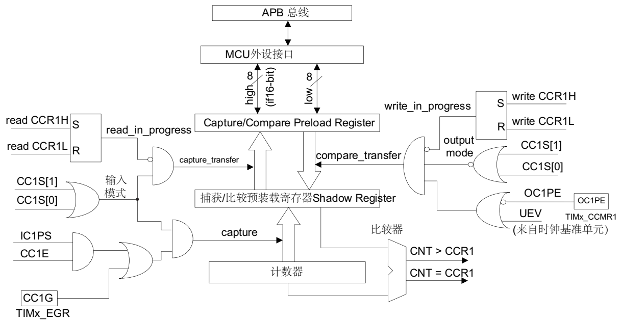
图 58. 捕获/比较通道 1 的主电路
