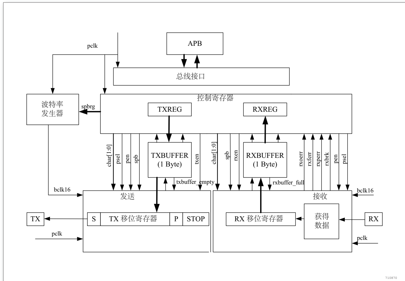
图 227. UART 方框图
