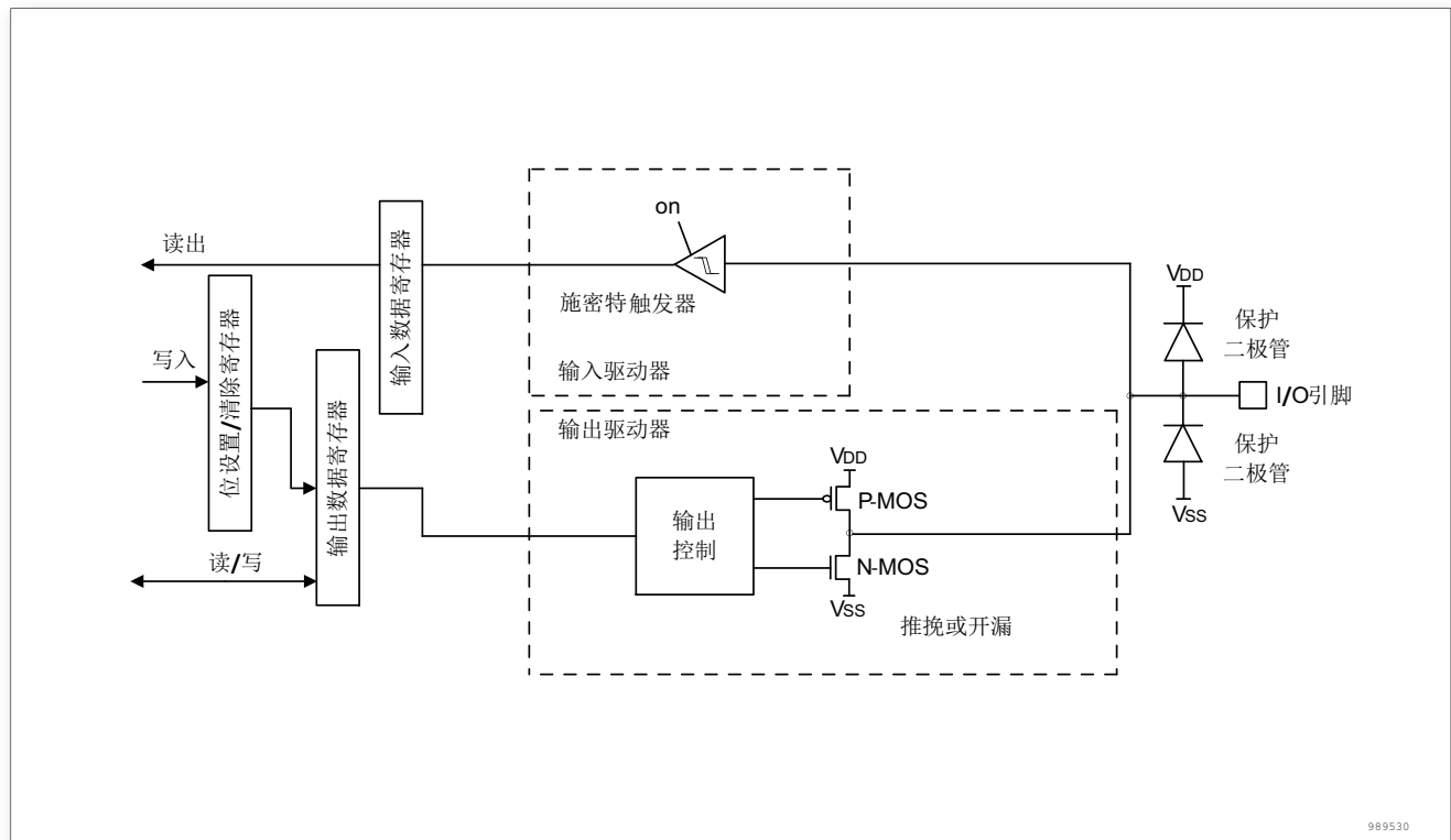
图 17. 输出配置
