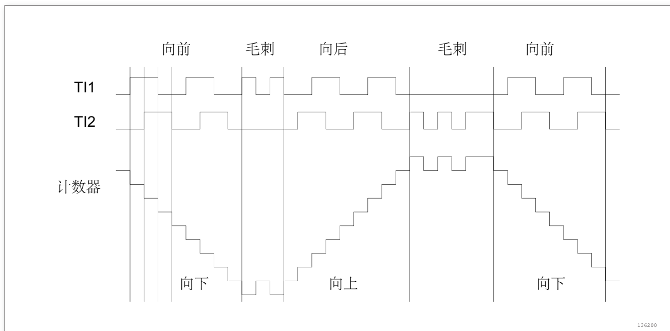
图 73. IC1FP1 反相的编码器接口模式实例
