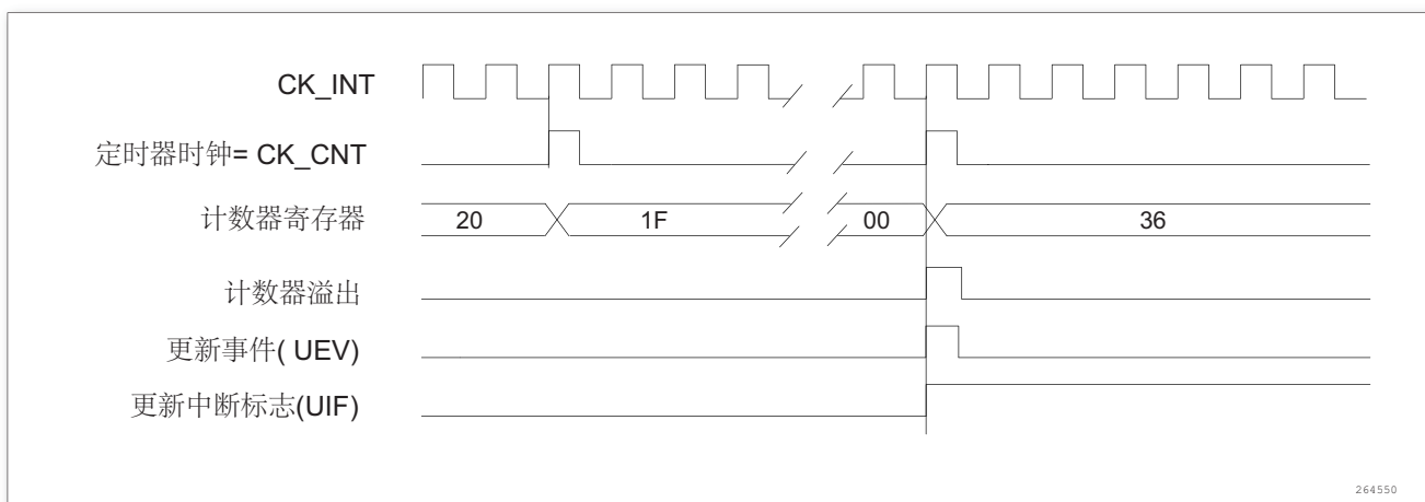
图 91. 计数器时序图，内部时钟分频因子为 N
