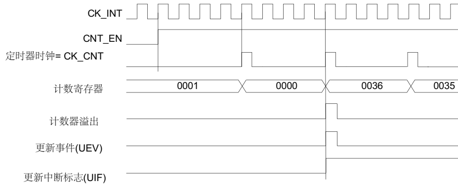
图 42. 计数器时序图，内部时钟分频因子为 4
